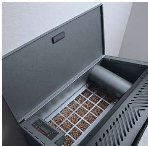
Pelletsförrådet rymmer hela 49 kg vilket motsvarar 240 kW/h. En normal villas genomsnittsförbrukning är 4 kW/h.
